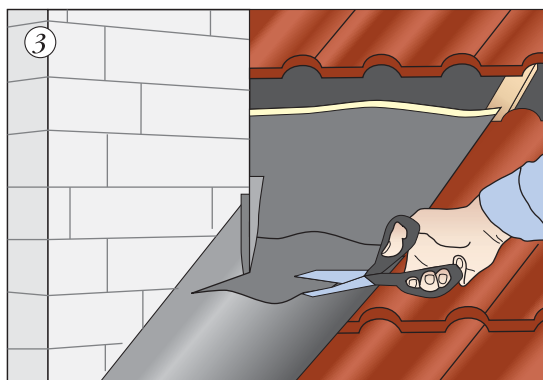
3 и низ углов
