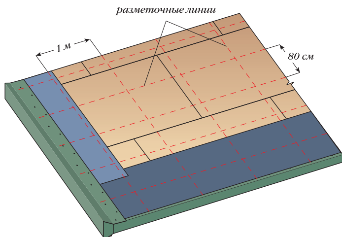
Рис. 124. Разметка ската
