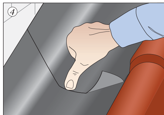
4 Приклеить Вакафлекс (все стыки должны быть сделаны по направлению стока воды)
