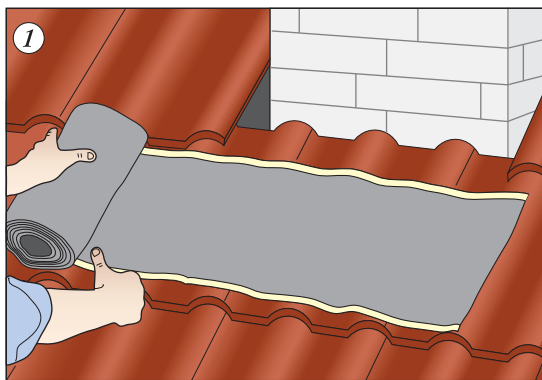
1 Отмерить и отрезать полосу Вакафлекса
