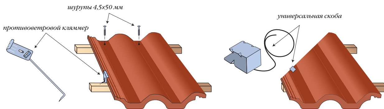
Рис. 51. Варианты крепления черепицы
