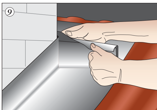
Установить верхнюю свинцовую полосу и соединить ее с боковой двойным фальцем
