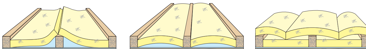
Рис. 12. Подготовка утеплителя к работе и его правильная укладка
