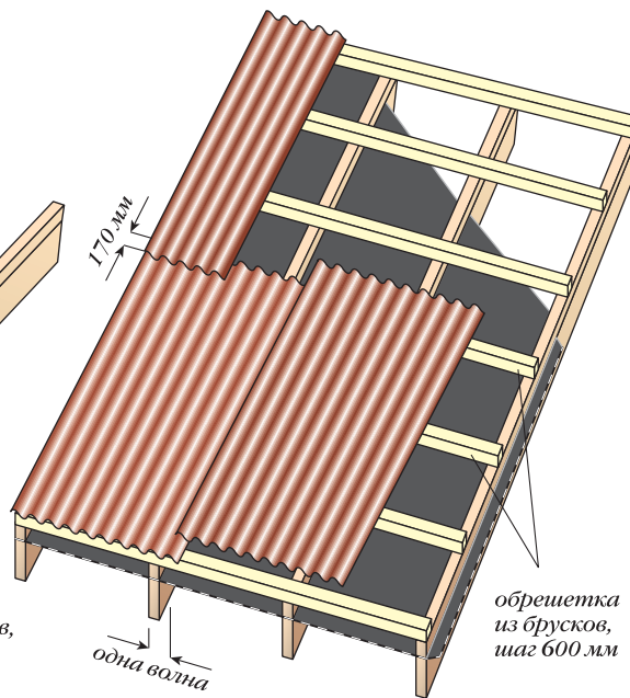
Наклон ската более 15°
