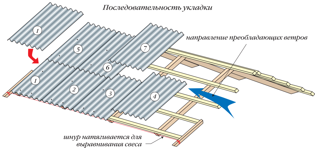
Рис. 27. Правила укладки шифера
