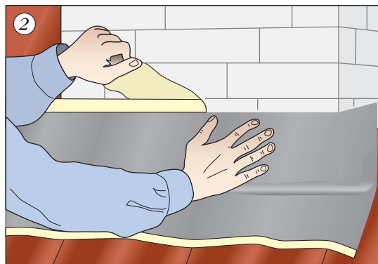
2 Наклеить ее сначала на трубу...
