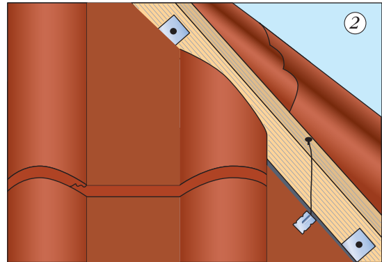
Черепицу крепить с зазором к бруску 20-30 мм, применяя при необходимости универсальные зажимы
