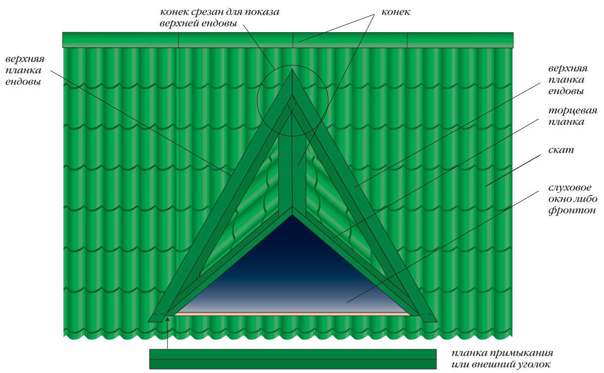
Рис. 80. Оформление коротких ендов
