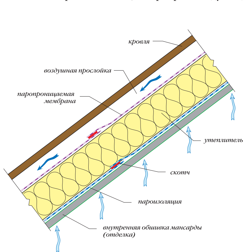
Рис. 19. Главный принцип нахлестов
