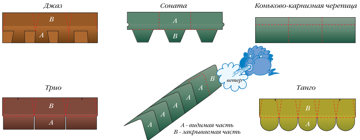
Рис. 133. Выкройка коньковых или хребтовых черепиц из рядовых
