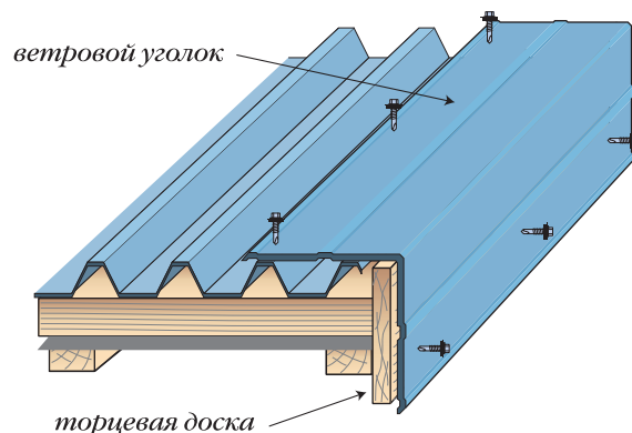
Рис. 86. Узел торцевого свеса крыши
