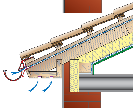
Рис. 52. Варианты узлов карнизного свеса: слева — с выносом стропила (кобылки) за стену; справа — без выноса
