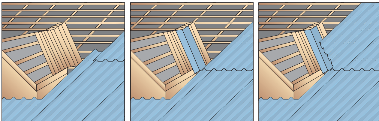
Установить нижние листы профнастила
