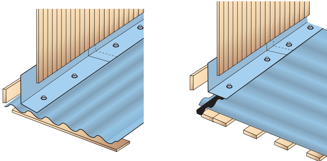
Рис. 91. Примыкания кровли к стенам
