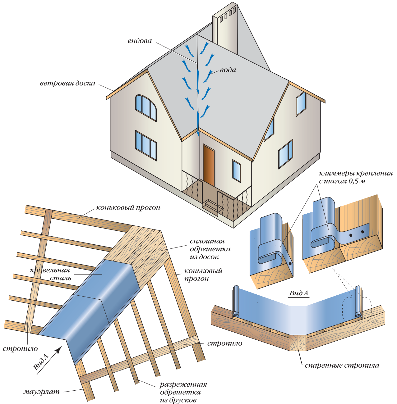
Рис. 5. Традиционное решение устройства узла ендовы
