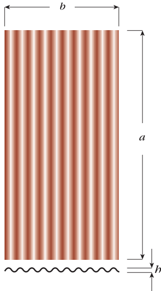
Кровельный лист
