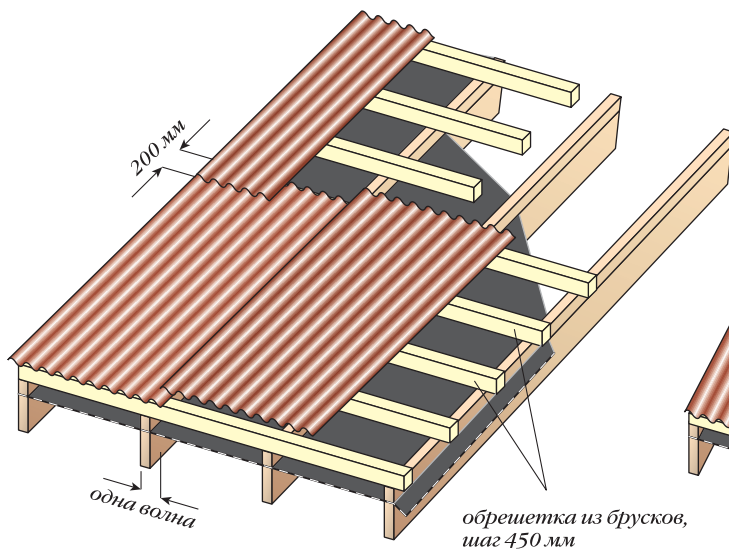
Наклон ската от 10 до 15°
