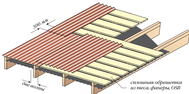
Наклон ската от 5 до 10°
