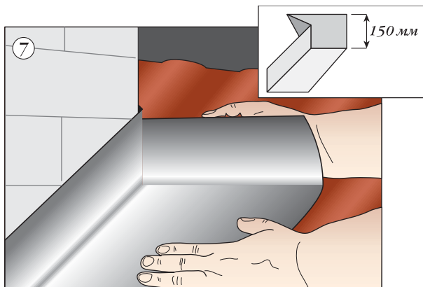
Верхний край свинцовой полосы загнуть на заднюю сторону трубы, соблюдая размеры
