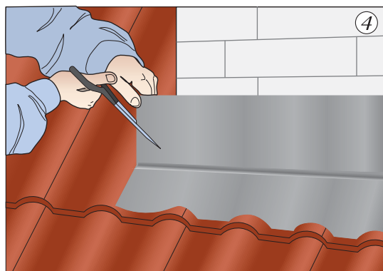
4 Подрезать углы и наклеить их на боковые стенки трубы
