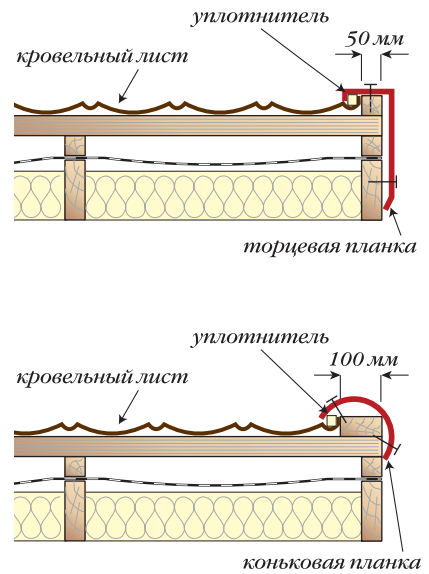
Рис. 103. Фронтонный свес кровли Roser
