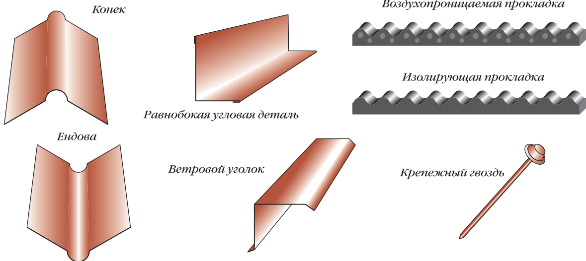
Рис. 28. Битумные волнистые листы и фасонные детали
